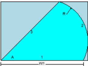
402SH - CONE (ANGLE&RADIUS)
