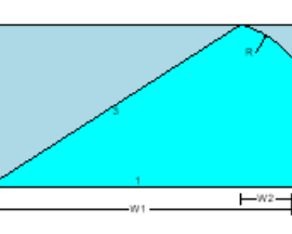
405SH - CONE RH (LEG, RADIUS&RISE)
